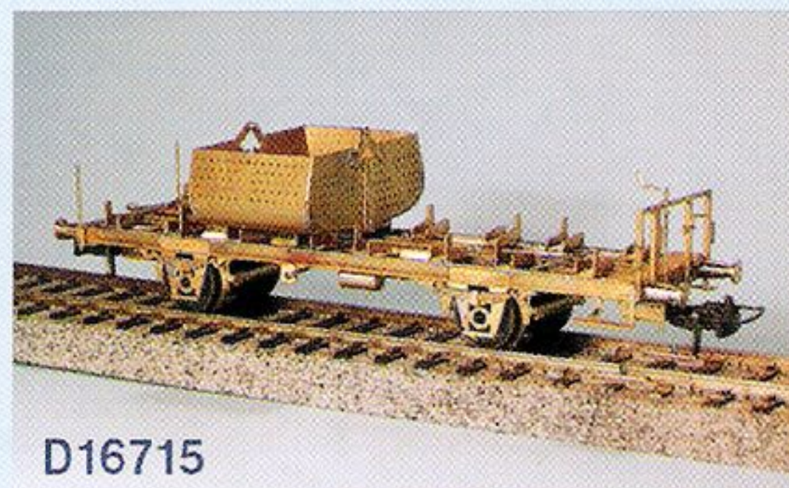
Brikettskübelwagen mit 4 Kübeln mit Bremsstelle
