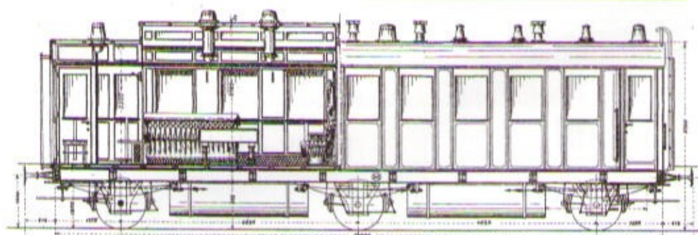
2.70.1 K.Bay.Sts.B. Salonwagen dreiachsig mit kompletter Inneneinrichtung abnehmbares Dach, feine Tampon - Linierung
