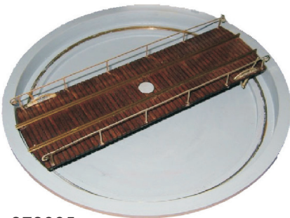
878005 12,8m drejeskive/Drehscheibe/turntable elektrisk drev, Electroantrieb/electric drive For AC and DC Spørlængde/ Länge der Bühne/length of tracks: 150 mm
