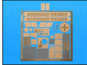
Instrumente, Lüftungsgitter
