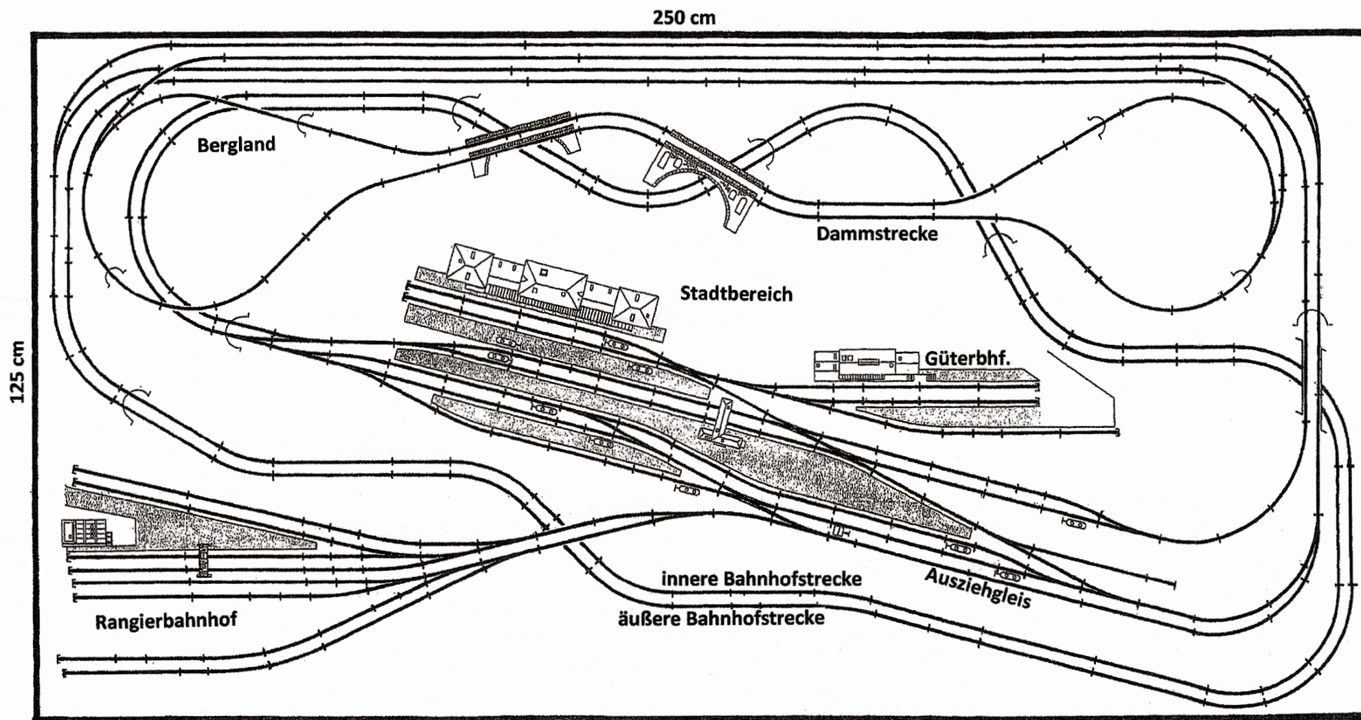
2,50 x 1,25 Meter: Der Übersichtsplan illustriert die Ausmaße unserer Anlage.
